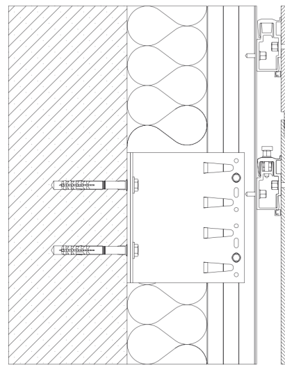
Przekrój systemu montażowego/ Cross-section of the installation system
