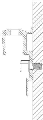
Przekrój elementu fasady Corian® wraz z zawieszem/ Cross-section of Corian® façade element including sling
