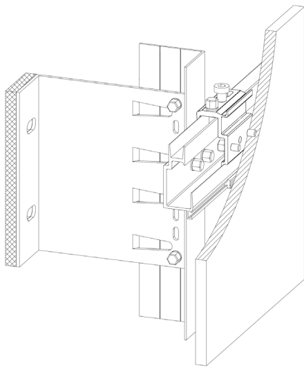
System montażowy wentylowanej fasady Corian®/ Corian® ventilated facade installation system
