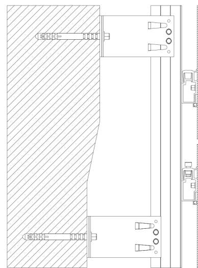
Przekrój systemu montażowego na nierównej powierzchni budynku/ Cross-section of the mounting system on an uneven building surface
